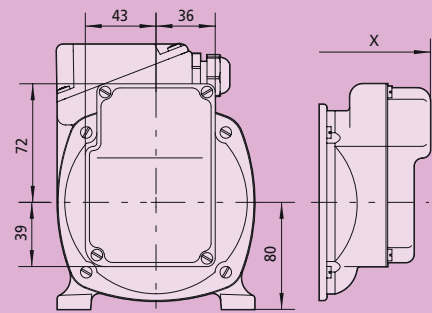
Frein à disque / Disk brake
