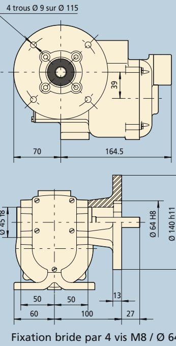
Modèle à bride B5 / Flange model B5 - Symbole -T-
