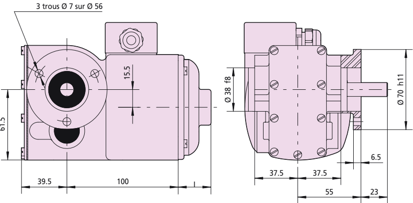
Fixation bride par 3 vis M5 / Ø 50
