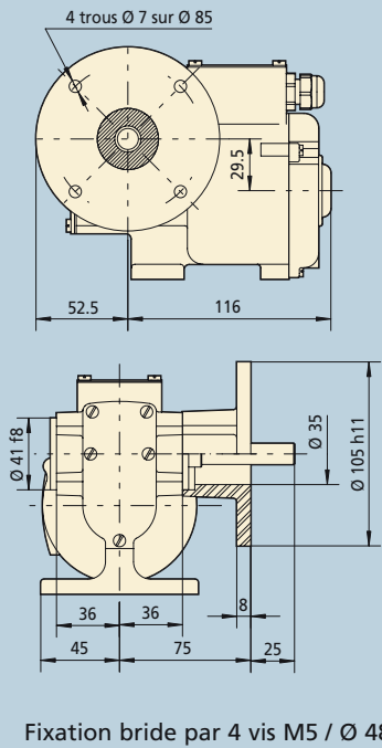
Modèle à bride B5 / Flange model B5 - Symbole -T-
