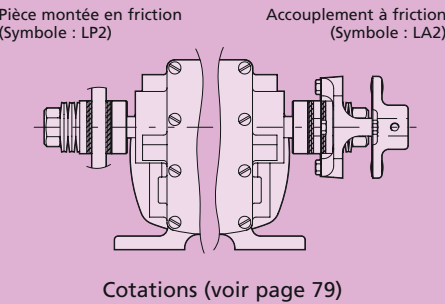
Cotations (voir page 79)
