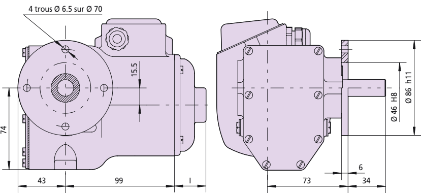
Fixation bride par 4 vis M6 / Ø 60
