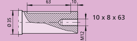
Clavetage / Keyway
