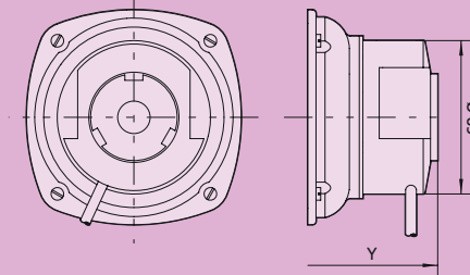
Frein à disque / Disk brake
