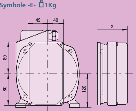
Frein à disque / Disk brake
